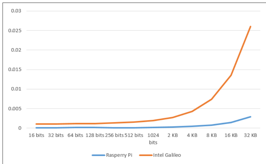
Figura 25 – Gráfico de deciptação AES para as plataformas Raspberry Pi e Intel Galileo utilizando chave de 256 bits
