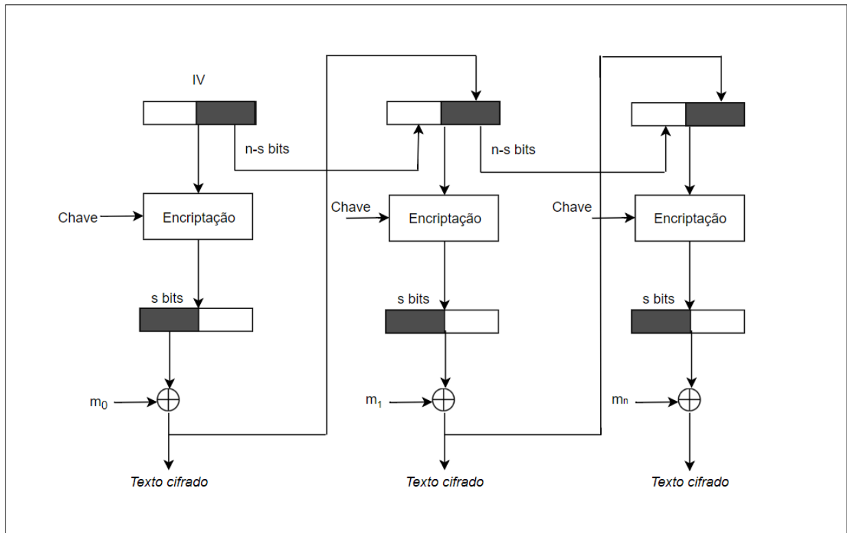
Figura 8 – Modo CFB
