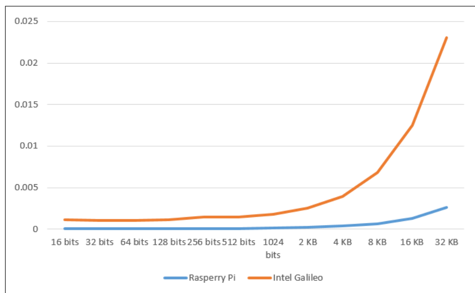
Figura 23 – Gráfico de deciptação AES para as plataformas Raspberry Pi e Intel Galileo utilizando chave de 128 bits
