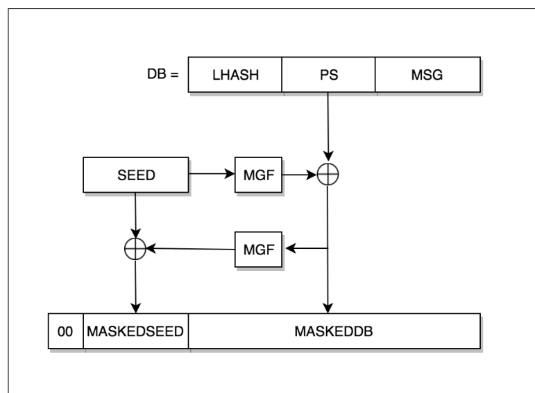
Figura 12 – Esquema OAEP
